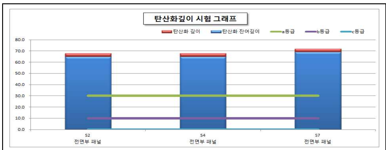
【그림 11.4.3】 탄산화 깊이 측정결과
